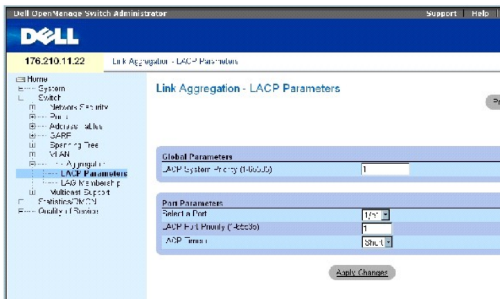
Figura 7-38. LACP Parameters
